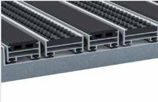
lastik + geniş fırça rubber+wide brush
